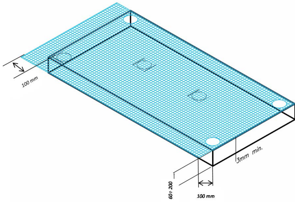
Figure 1 : Panneau Ecap
