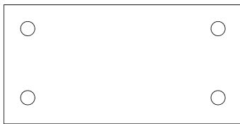
Panneau standard usine 4 chevilles/ panneau – 8 chevilles / m 2
